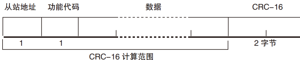
图 9-3 异常响应帧
